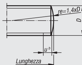
LD Perno lungo
