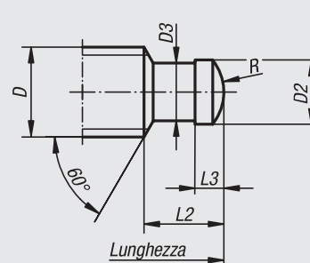
Estremità a norma DIN 6332
