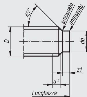
TC Punta, appiattita
