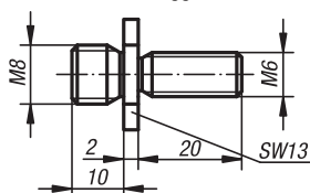
Adattatore di fissaggio M8/M6
