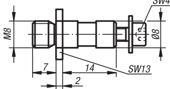
Adattatore di fissaggio M8/Ø8
