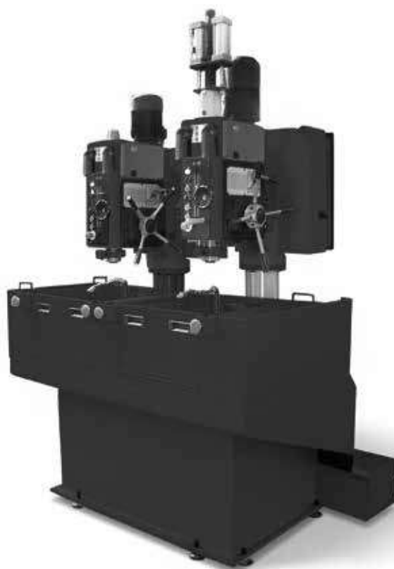
Batería de 2 unidades (taladrado-roscado por husillo patrón) para rótulas de automoción.
